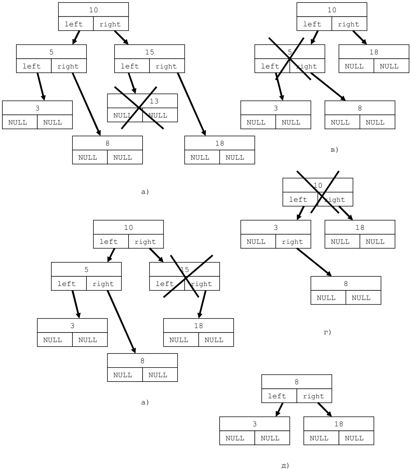
Рисунок 11 - Исключение узлов из дерева
