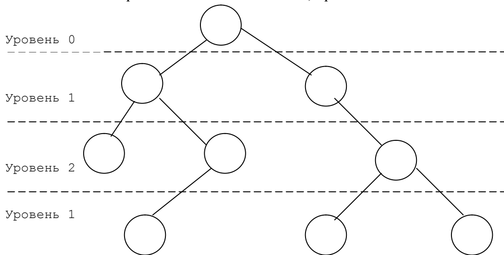
Рисунок 8 – Бинарное дерево
